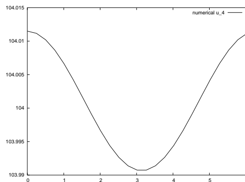
Figure 6: Solution exacte/approchée u_3 Solution approchée u_4
