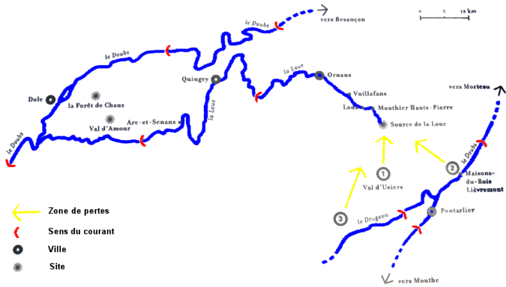
Figure 15: Schéma résurgence du Doubs
